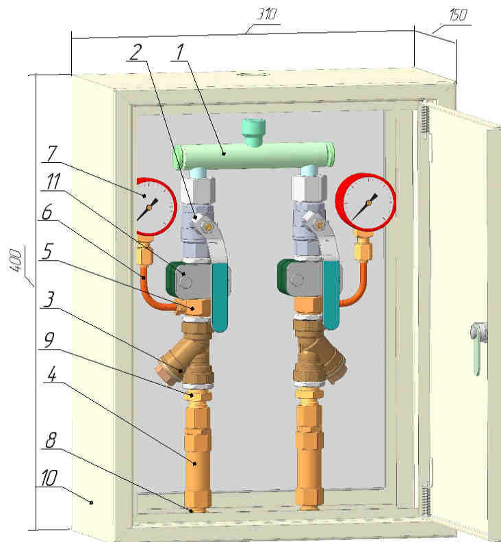
Рис. 1. Пост газоразборный ПГГ-10з-2
